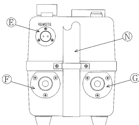
右側面図
